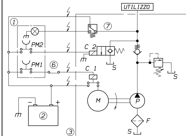
Schema di collegamento MOTORE-TELERUTTORE/Motor-remote control switch connection diagram
